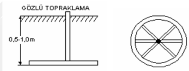
Şekil 18 Gözlü Topraklayıcı [58, s10]
