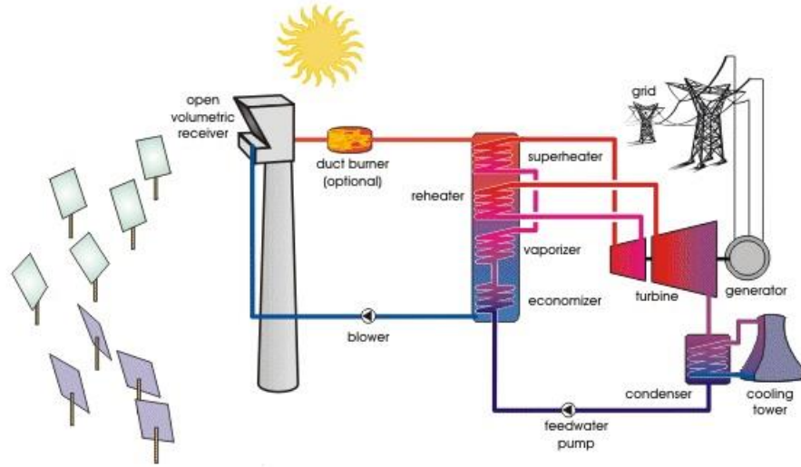
Şekil 9 Termal Güneş Enerjisi Santrali [48]
