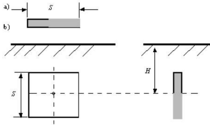
Şekil 21 Kare Topraklayıcı [56, s94]
