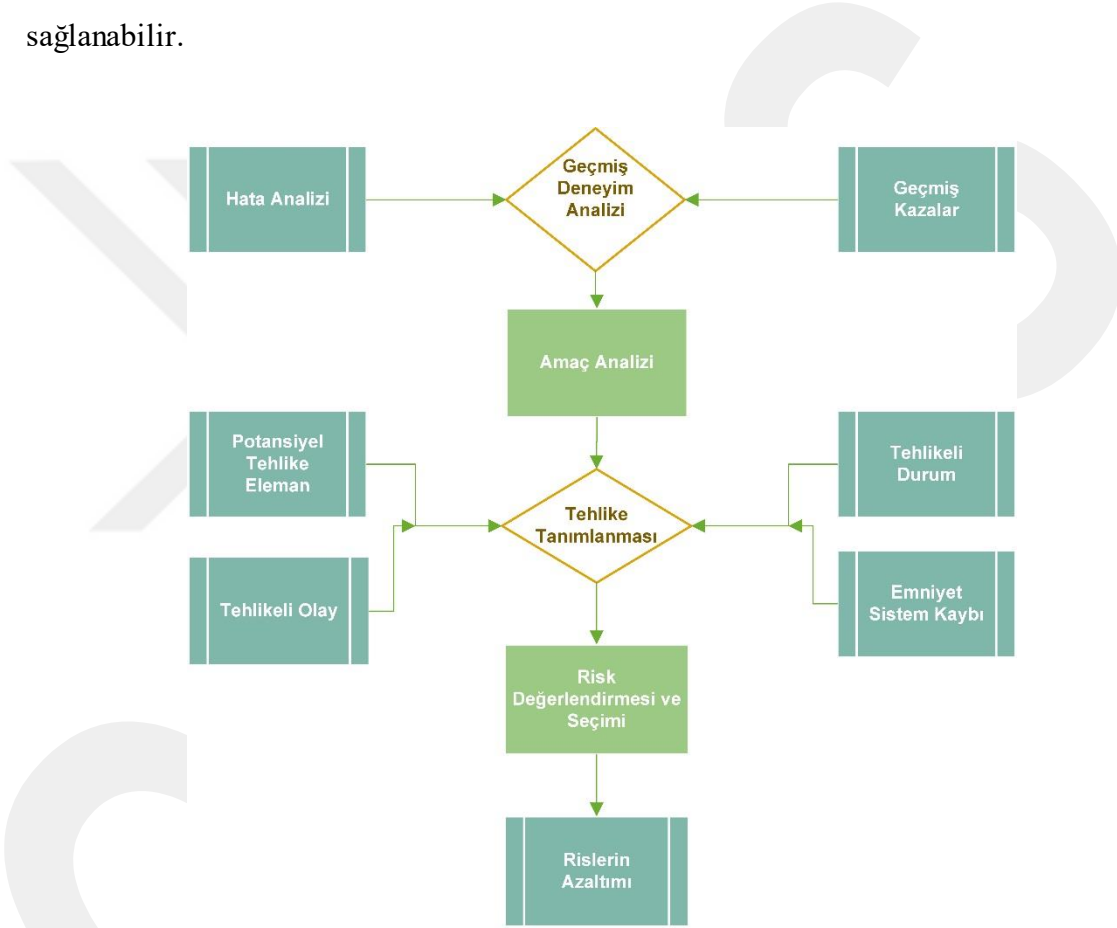
Şekil 4 Ön Tehlike Analizinin Çalışma Yöntemi [31,s117]
