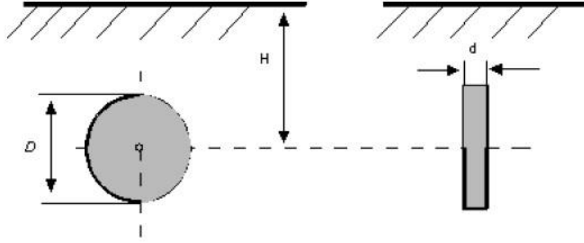
Şekil 20 Düşey Gömülen Topraklayıcı [56, s93]
