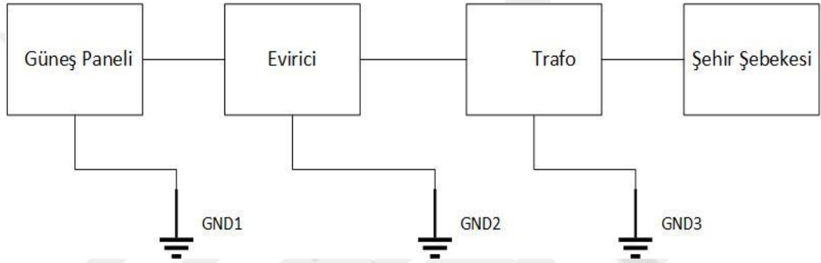
Şekil 19 Çubuk Topraklayıcılar[58,s10]
