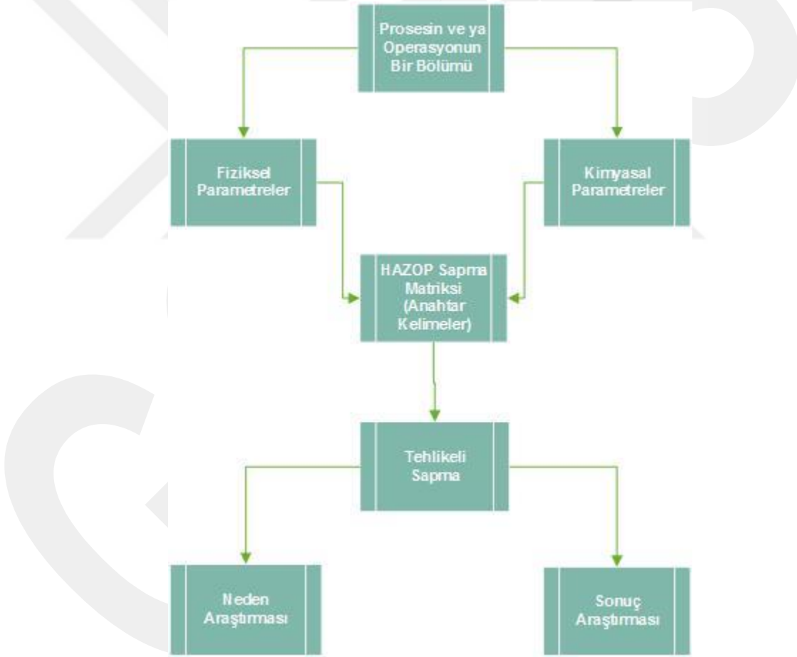
Şekil 5 HAZOP Tehlike Saptama Hipotezi [31, s140]
