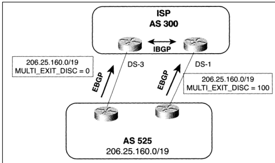
Figure 17. MED Attribute [6]
