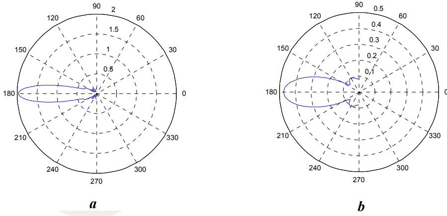
Şekil 5: (\rho_0:0.3m, \phi_0:0, \phi_{01}:\pi/3; \rho_0:1m, \phi_0:\pi, \phi_{01}:\pi/6) için ışın diyagramları
