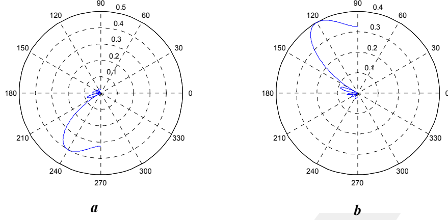
Şekil 4: (\phi_0:2\pi/3; \rho_0:0.5m) ve \phi_0:4\pi/3, \phi_{01}:\pi/4 için ışın diyagramları
