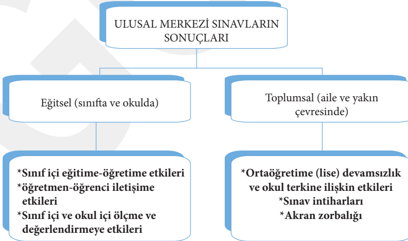
Şekil 2. Ulusal Merkezi Sınavların Olası Sonuçları
